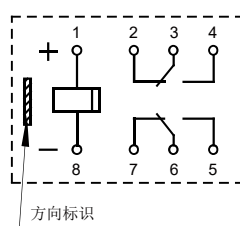
单稳态
