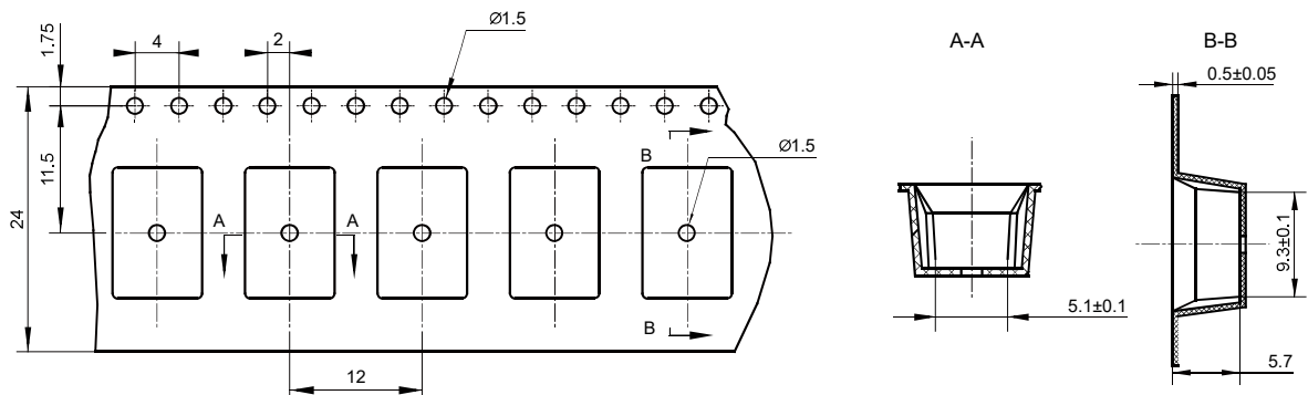
载带外形图
