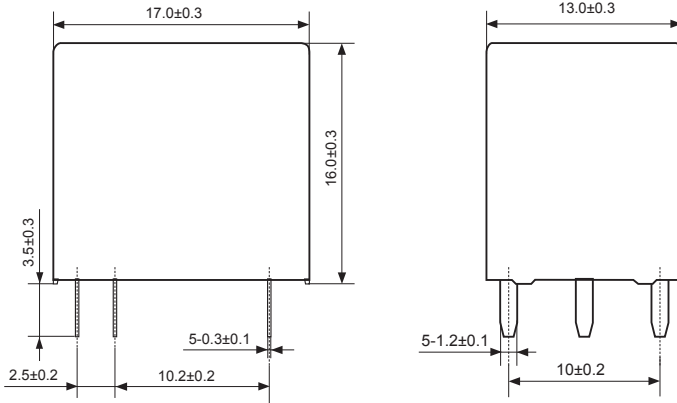
外形图
